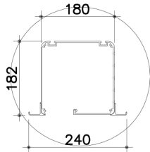
AL case
